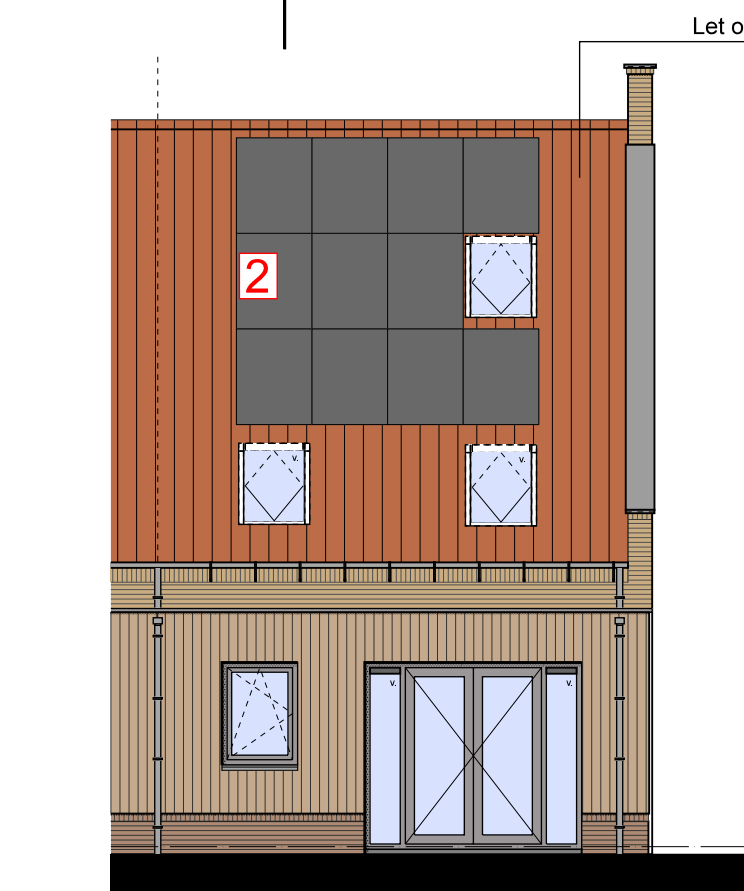
ACHTERGEVEL
