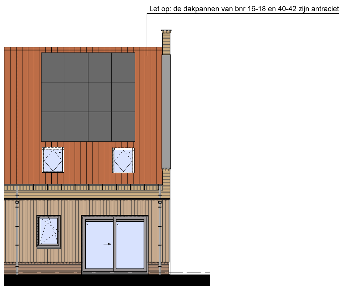
4 ACHTERGEVEL
