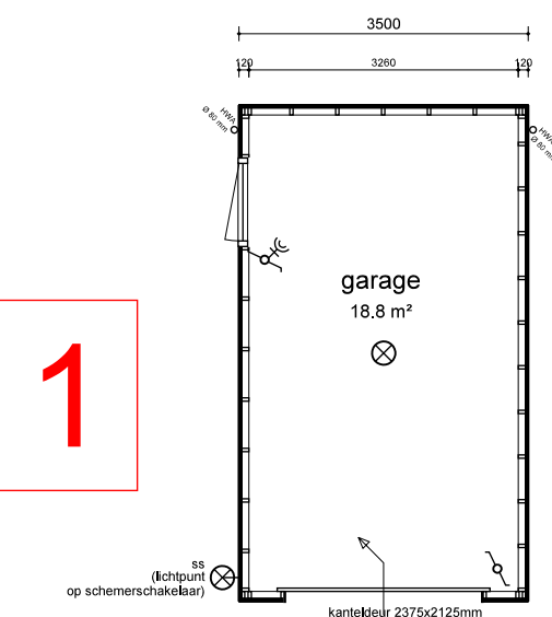
1 PLATTEGROND nummer 23, 24, 40, 42 nummer 41 als gespiegeld
