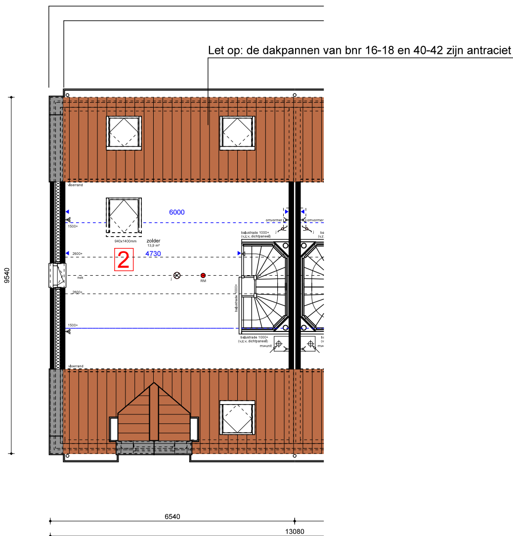
ZOLDER (optie 2)
