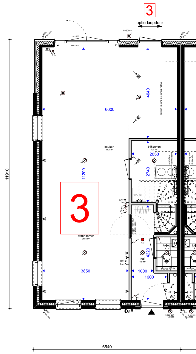
BEGANE GROND (optie 3)
