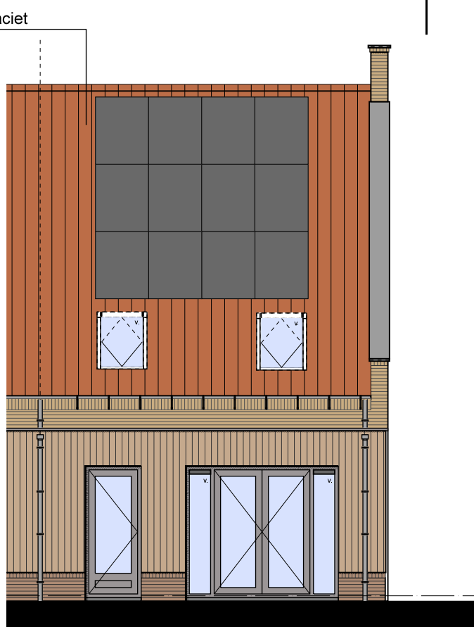
ACHTERGEVEL
